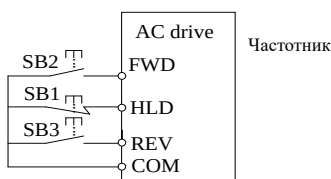
Рис.6-15 Трехпроводной режим управления 1
