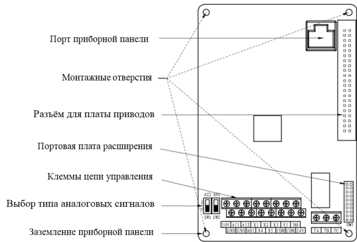
Рис. 3-20 Плата управления
