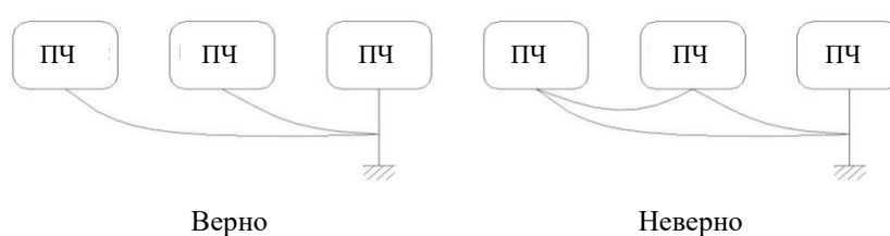
Рис. 3-5 Заземление
