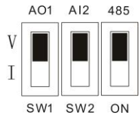
Рис. 3-21 Настройка двухпозиционного переключателя
