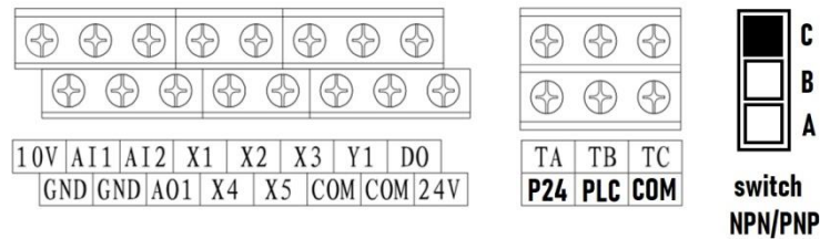
Рис. 3-10 Расположение клемм цепи управления для версии B2_0102
