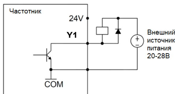
Рис.3-17 Способ подключения внешнего источника питания
