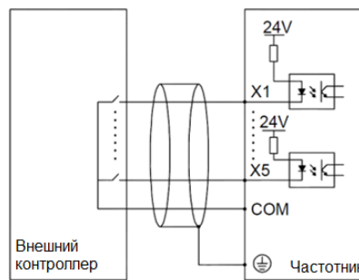
Рис. 3-11 Схема подключения цепи управления
