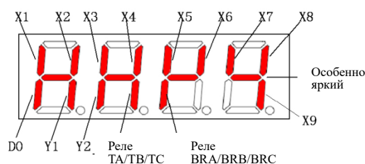
Рис. 6-28 Схема отображения текущего состояния статус клемм
