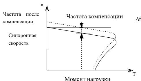
Рис. 6-11 Автоматическая компенсация скольжения
